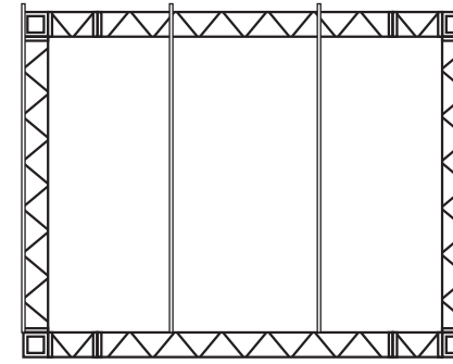
屋根伏図
